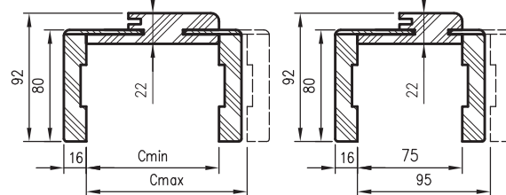
Průřez ORB
